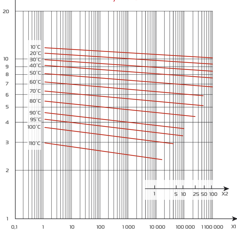
ДІАГРАМА ТЕРМІНУ ЕКСПЛУАТАЦІЇ PE-RT/EVOH
