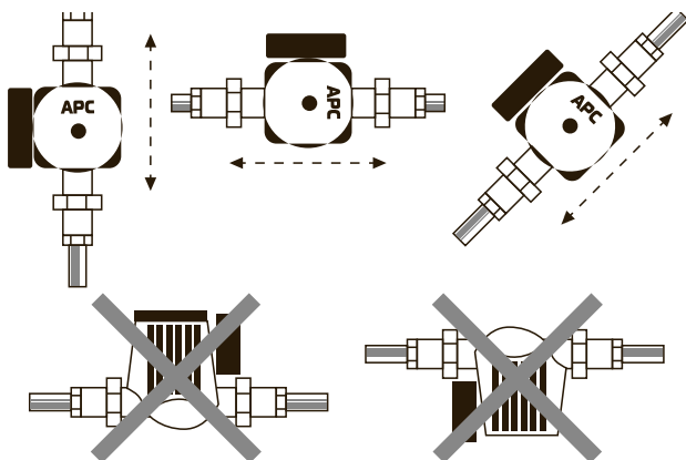
Рис. 2. Монтаж насоса на трубопроводе
