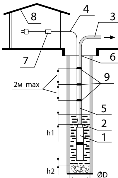
Рис.3 Схема монтажа насоса
