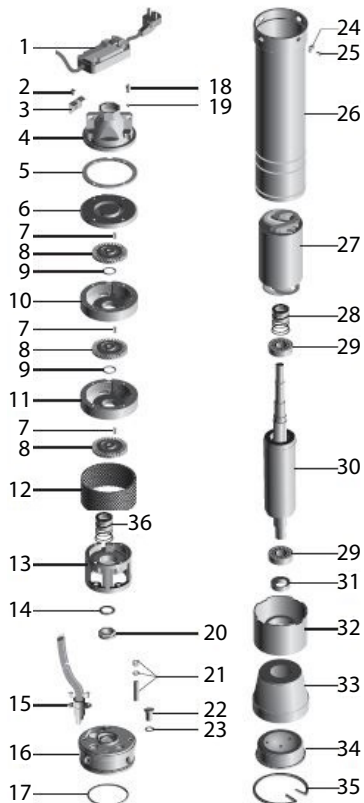
На рис. 1 изображена детальная схема насоса SKM
